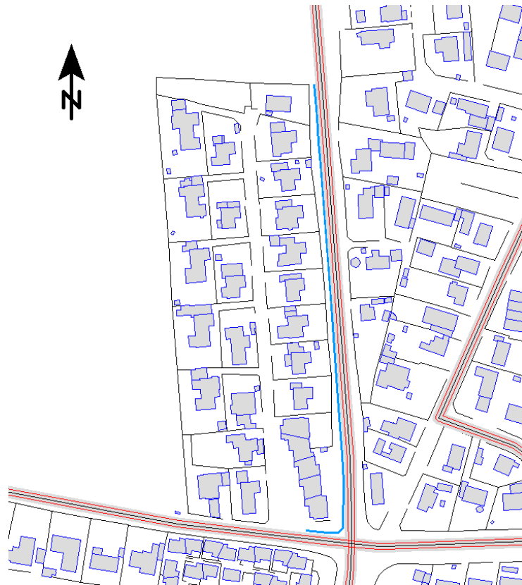
Figur 27: Figuren viser placeringen af de forslåede støjskærm langs med Hillerødvej i Lyngby. Støjskærmen er vist med blåt.
