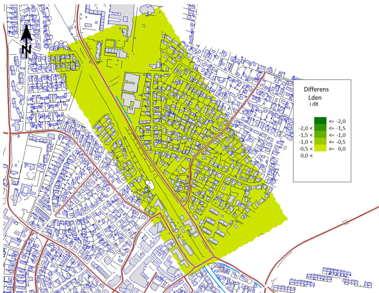
Figur 24: Differens kort. På figuren ses effekten af den støjreducerende belægning. Beregningshøjde 1,5 m over terræn.
